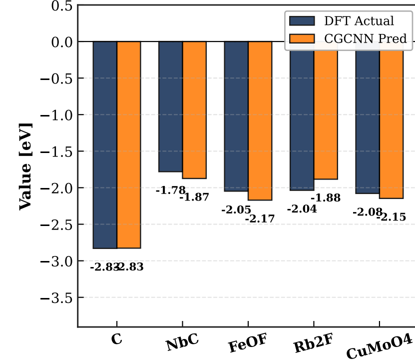
(d) Li Adsorption ( E_{\text{ads}} )
